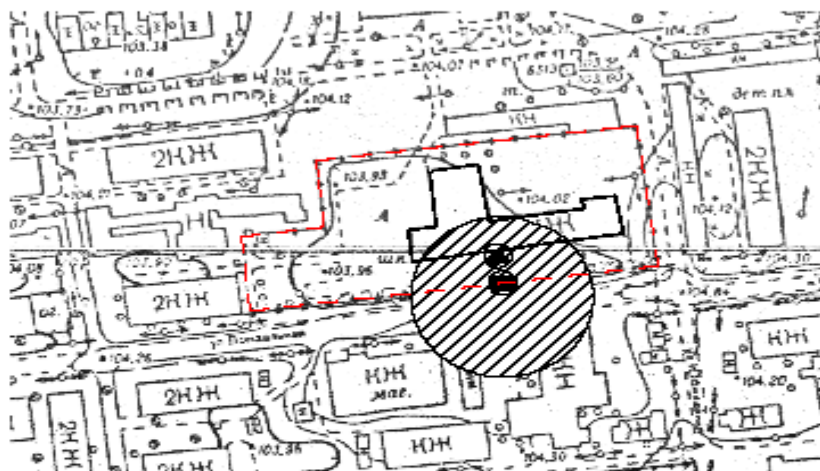
Схема генерального плана
