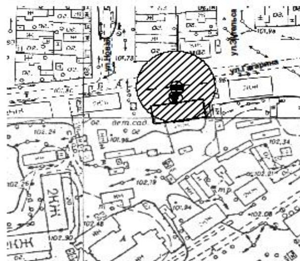
Схема генерального плана
