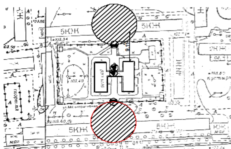
Схема генерального плана
